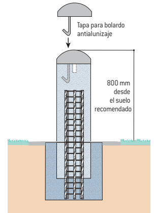
■ Ref. 206445 ø 273 mm
